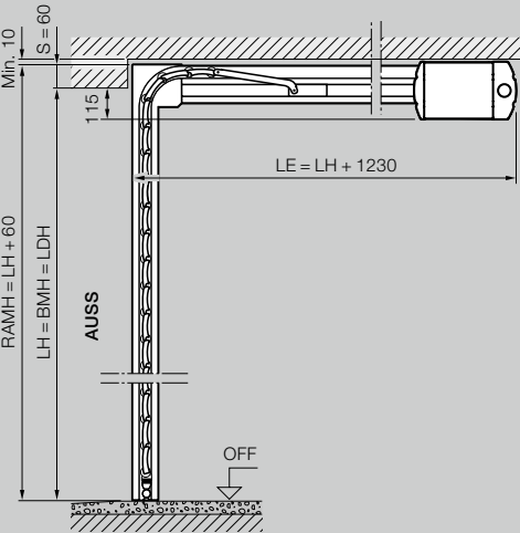
Maatbereik garagedeur RollMatic OD
