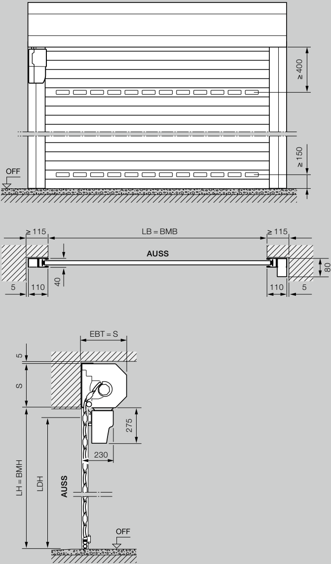
Maatbereik binnen- en buitenroldeuren
